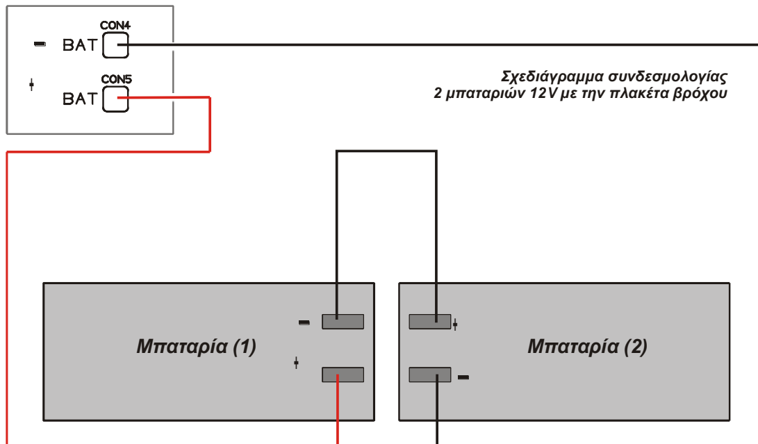
Σχήμα 4-4. Σύνδεση μπαταριών σε σειρά.
