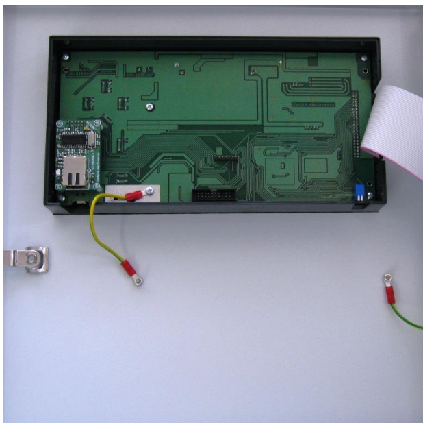
Σχήμα 4-2. Εσωτερικό πίνακα
