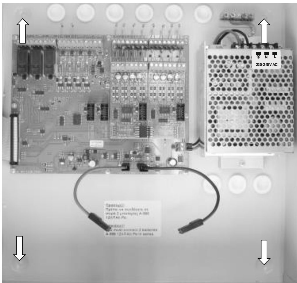
Σχήμα 4-1. Οπές στήριξης του πίνακα.
