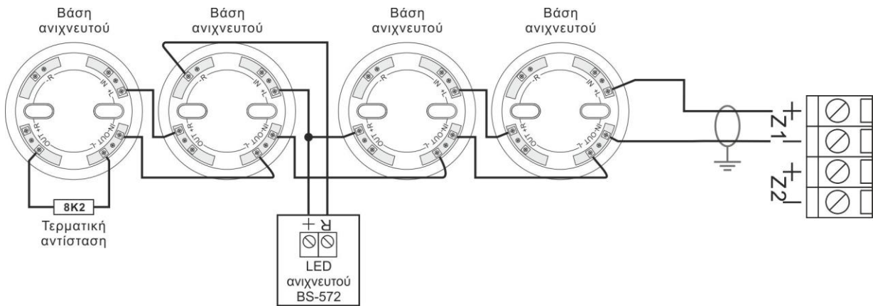
Σχήμα 4-5. Σύνδεση 4 βάσεων ανιχνευτών στη ζώνη 1. Στην κάθε βάση μπορεί να τοποθετηθεί ανιχνευτής BS-655, BS-660 ή BS-657. Σε έναν ανιχνευτή είναι συνδεδεμένο ένα LED ανιχνευτή BS-572.
