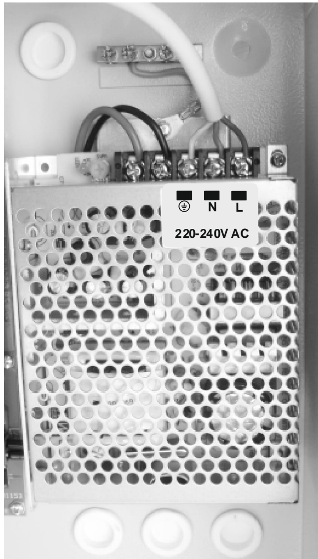
Σχήμα 4-3. Σύνδεση 230VAC
