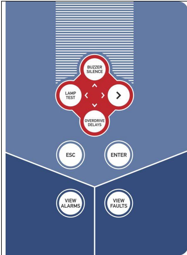
Σχήμα 1-2. Πληκτρολόγιο πίνακα
