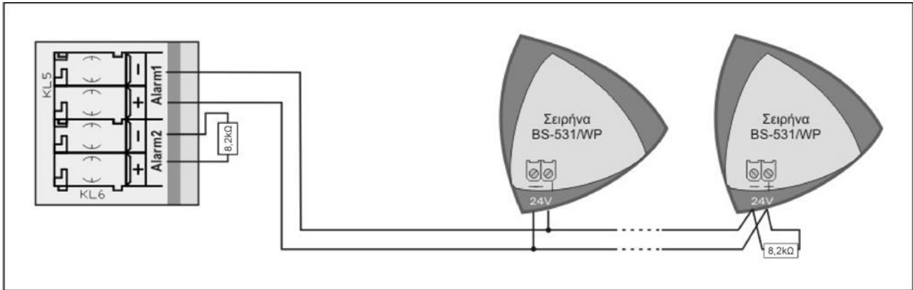
Σχήμα 4-8. Σύνδεση σειρήνων στον πίνακα
