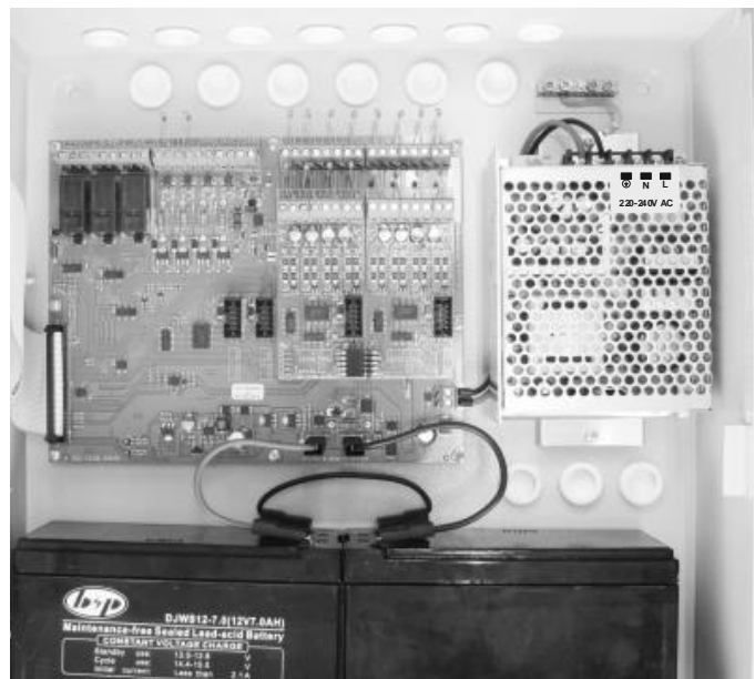
Σχήμα 4-2. Εσωτερικό πίνακα
