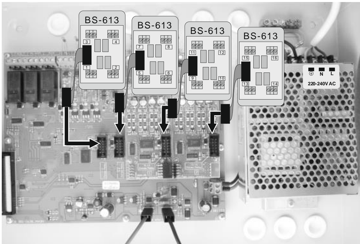
Σχήμα 4-9. Σύνδεση συσκευών BS-613.
