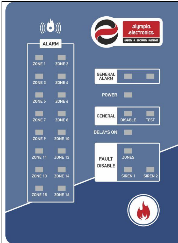
Σχήμα 1-3. Ενδεικτικά LED
