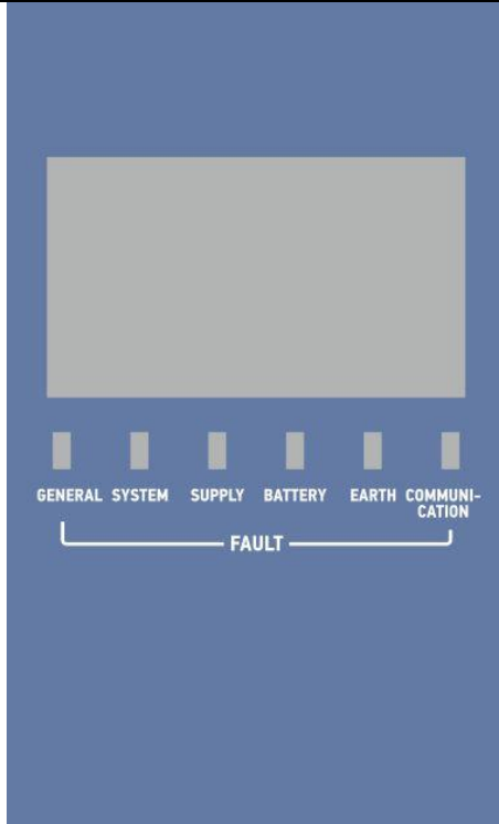
Σχήμα 1-4. Ενδεικτικά LED κάτω από την οθόνη
