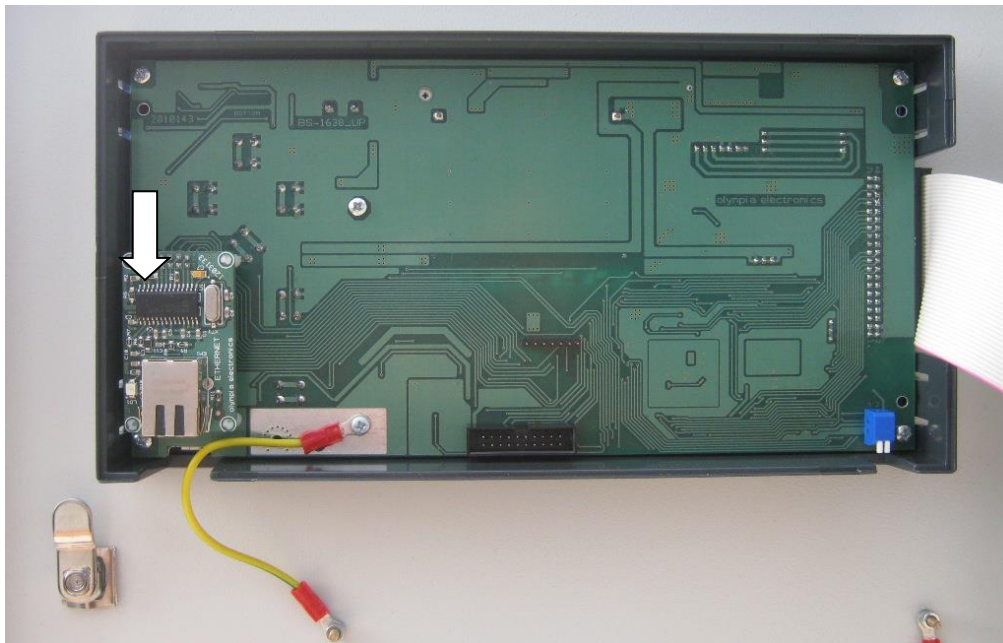
Σχήμα 4-10. Τοποθέτηση Ethernet
